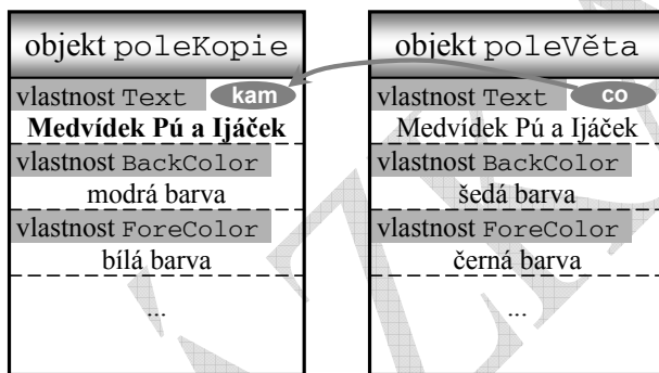
Obr. 29 Objekty po realizaci přiřazení
