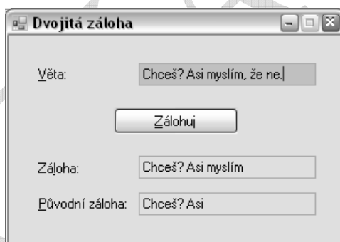
Obr. 31 Program ilustrující otázku sekvenčního zpracování
